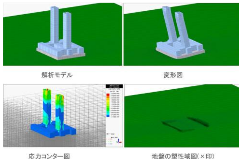
橋梁下部工の地震応答解析例
