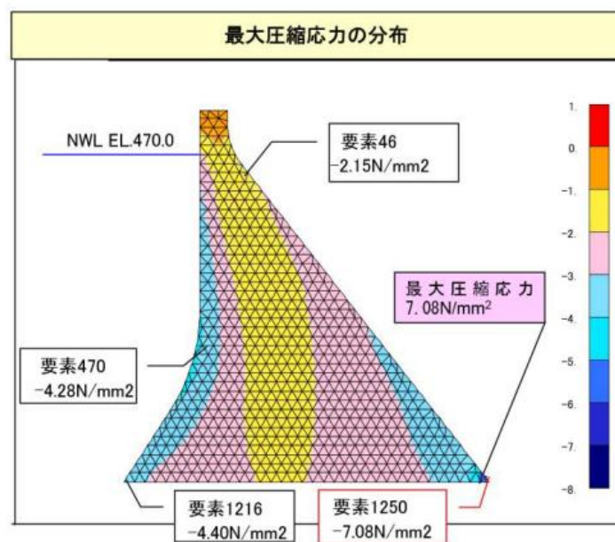
コンクリートダム地震応答解析例
