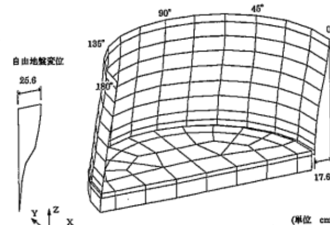
自由地盤と側壁の変位分布
