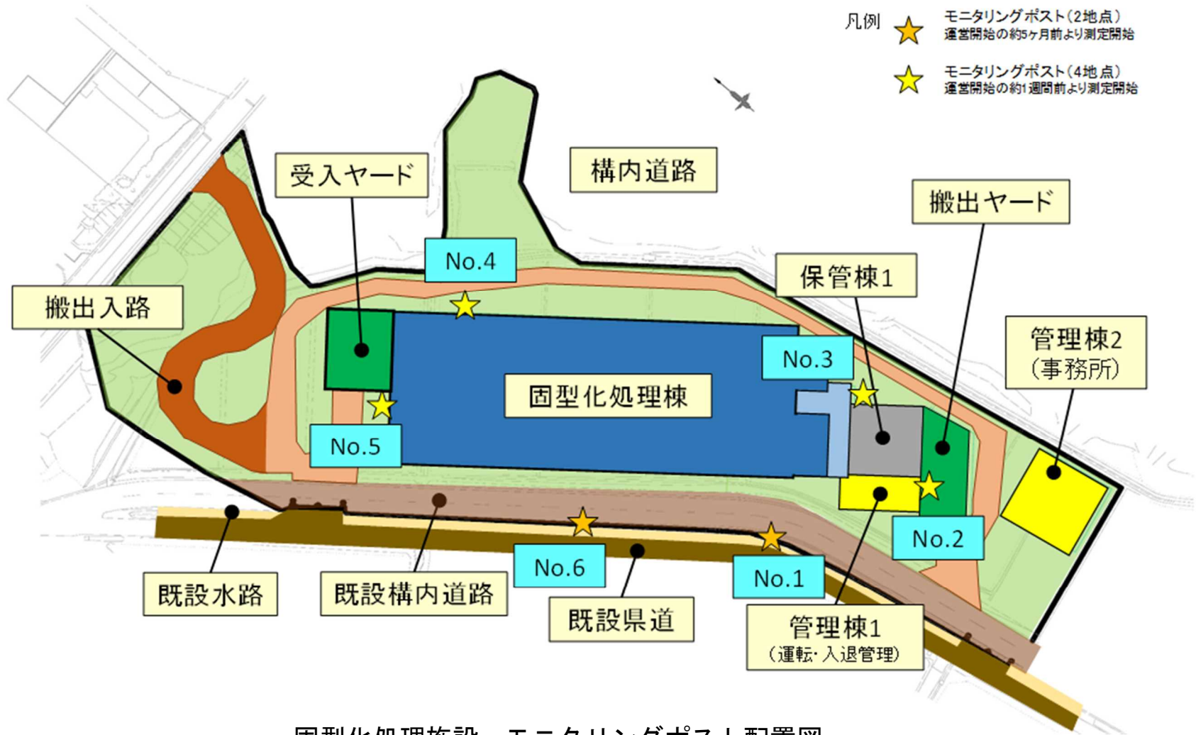
固型化処理施設 モニタリングポスト配置図
