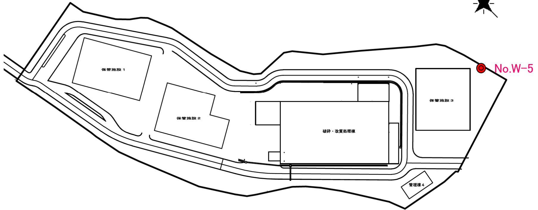
破碎・改質処理、第四保管施設 観測井位置図
