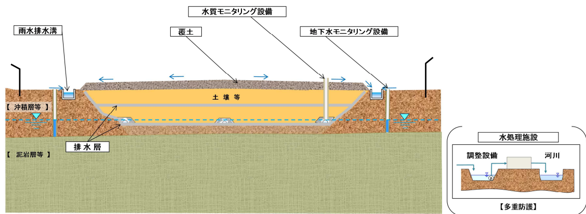
図4 土壌貯蔵施設（Ⅰ型）の構造等のイメージ（貯蔵時）
