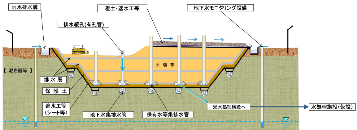
図5 土壌貯蔵施設（Ⅱ型Aタイプ）の構造等のイメージ（搬入時）
