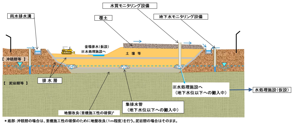
図3 土壌貯蔵施設（Ⅰ型）の構造等のイメージ（搬入時）
