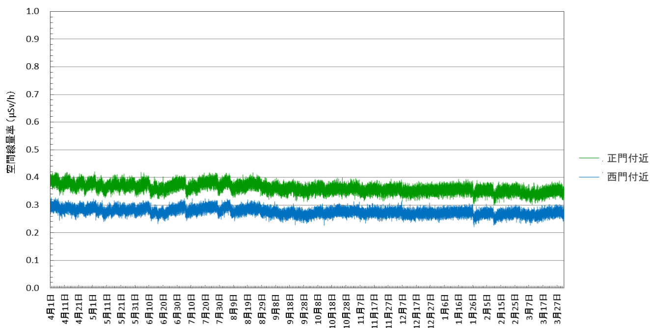
図 3-3-2 空間線量率(連続測定)の経時変化 (平成 30 年 4 月～平成 31 年 3 月)
