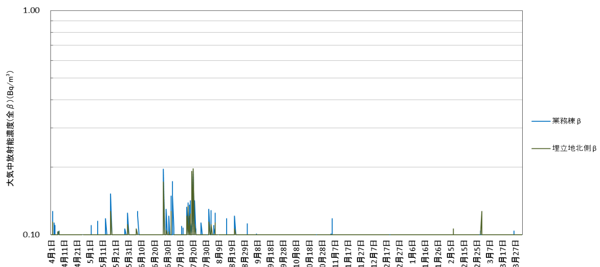
図 3-2-2 (2) 大気中放射能濃度(全 \beta )の経時変化(平成 30 年 4 月～平成 31 年 3 月)
