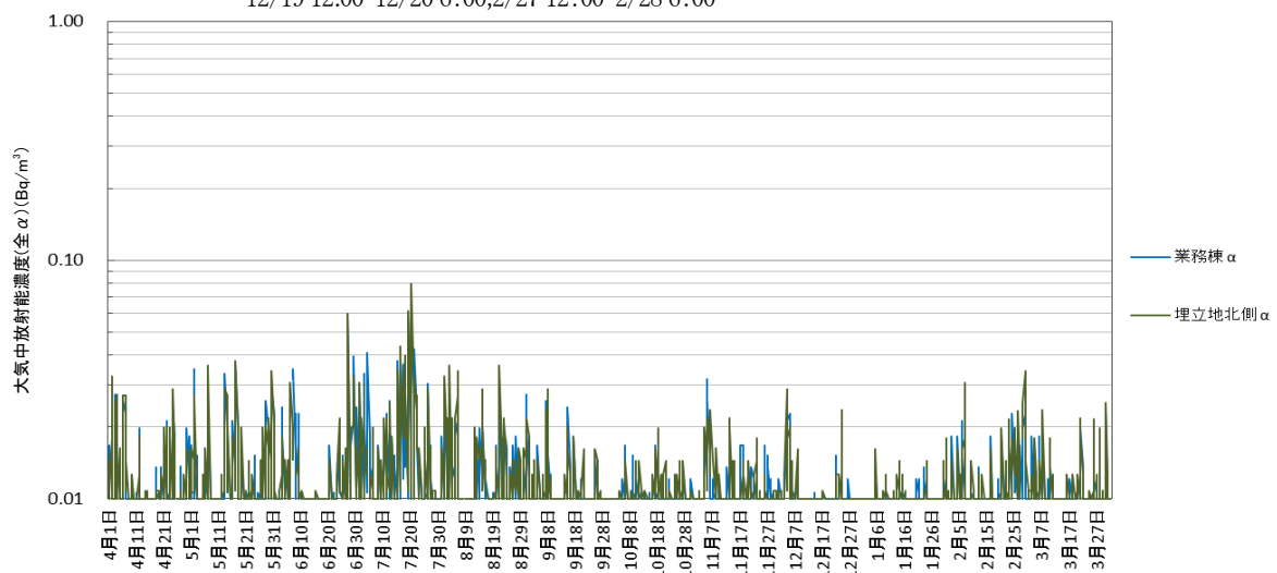
図 3-2-2 (1) 大気中放射能濃度(全 \alpha )の経時変化(平成 30 年 4 月～平成 31 年 3 月)
