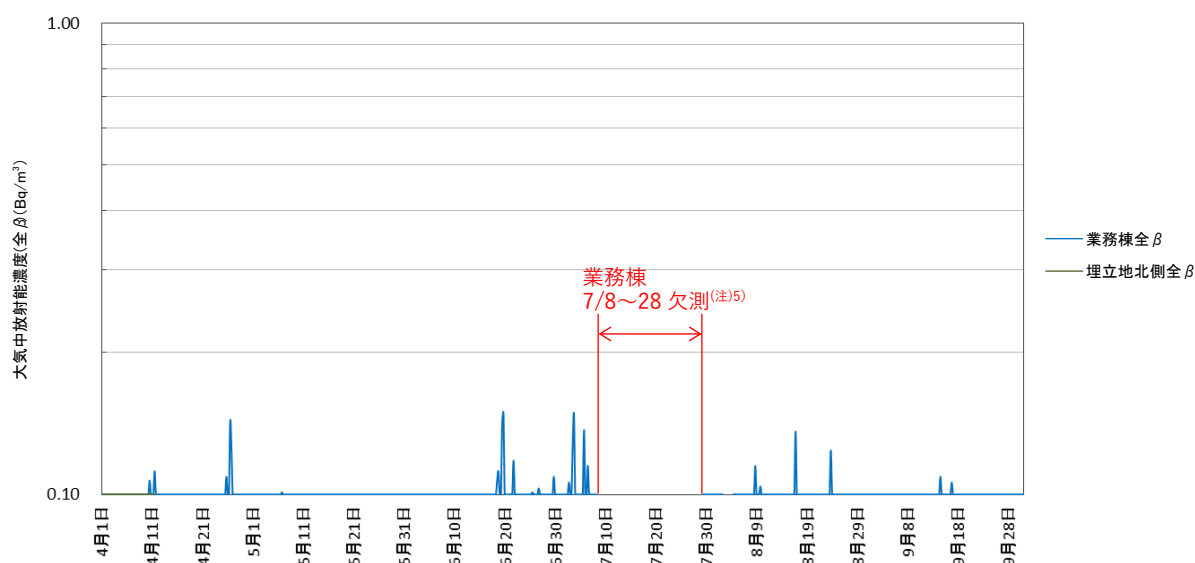
図 3-2-2 (2) 大気中放射能濃度(全 \beta )の経時変化(令和4年4月~9月)
