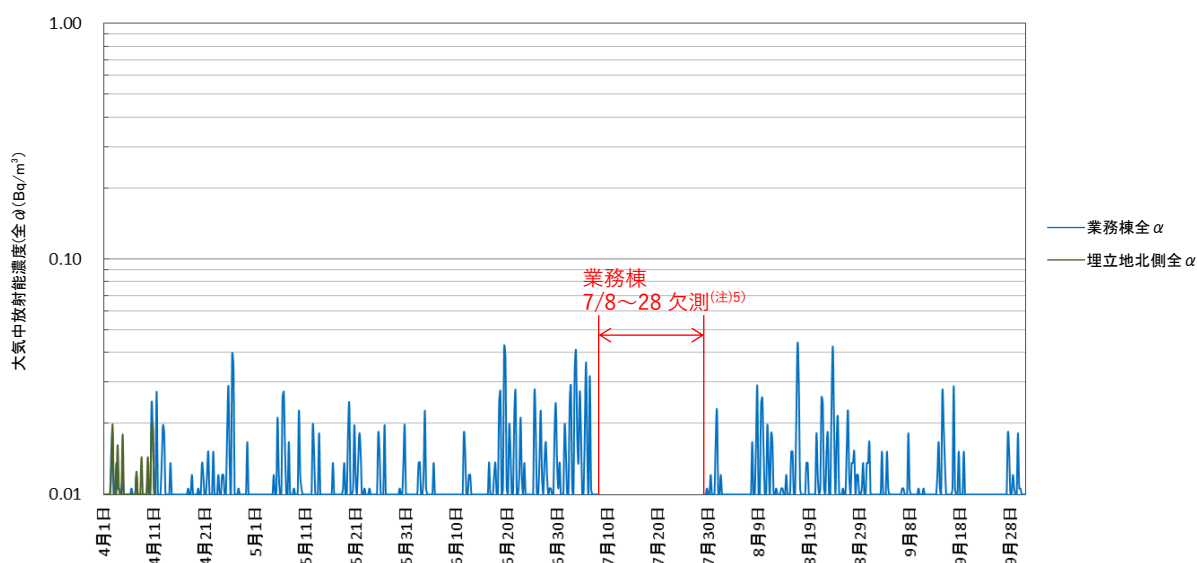
図 3-2-2 (1) 大気中放射能濃度(全 \alpha )の経時変化(令和4年4月~9月)
