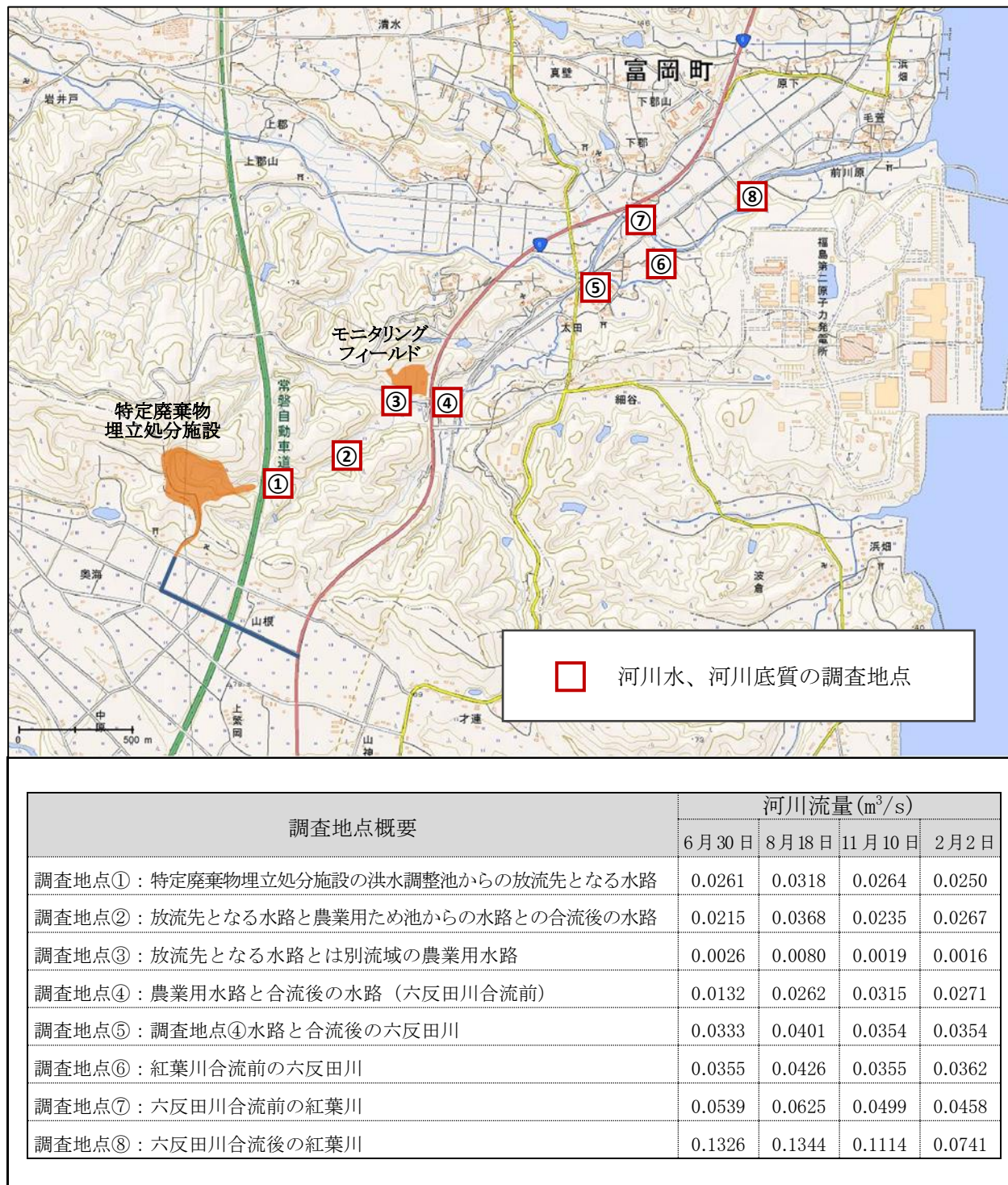
図 2-10-1 河川水、河川底質の調査地点及び河川流量
