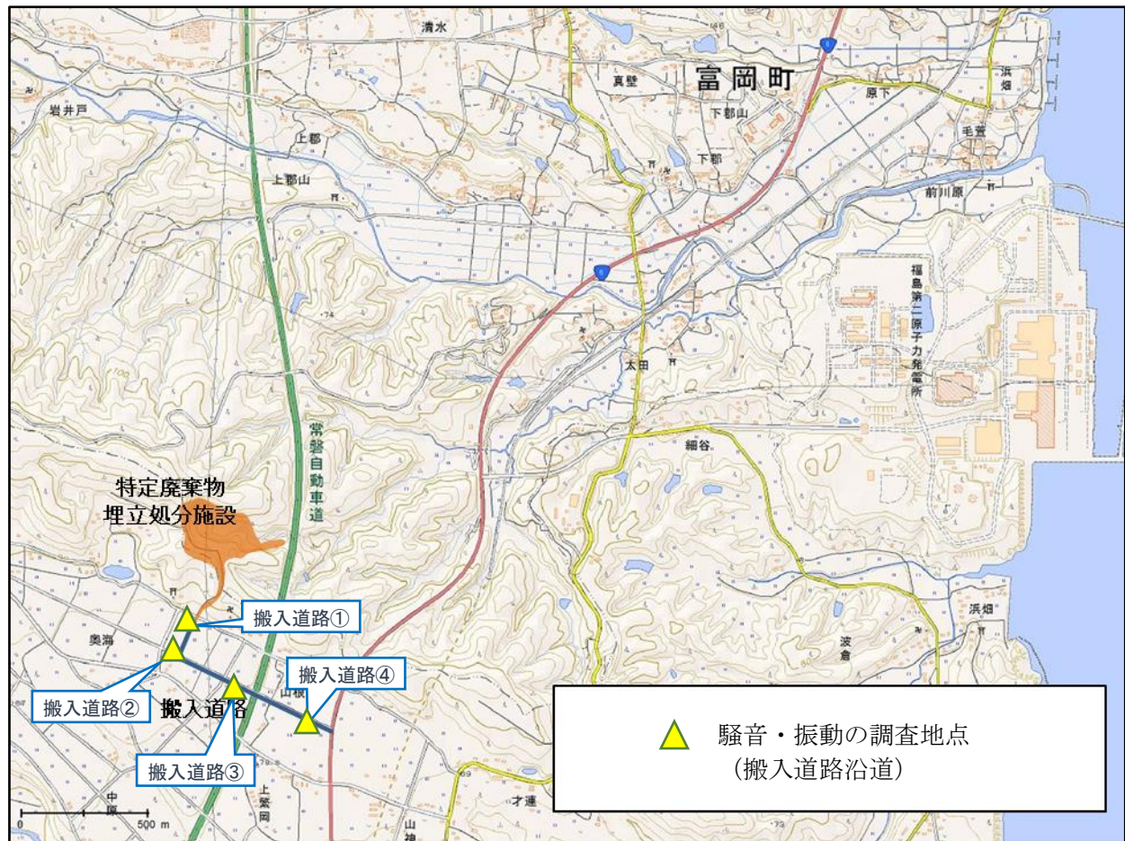
図 2-8-2 騒音・振動の調査地点 (搬入道路沿道)
