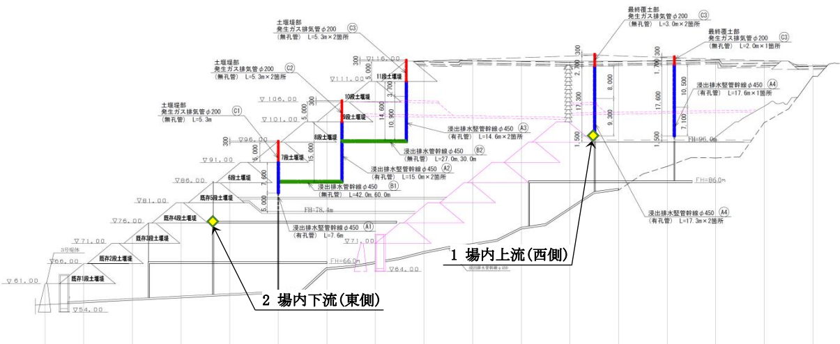
図 2-9-2 埋立ガスの調査位置
