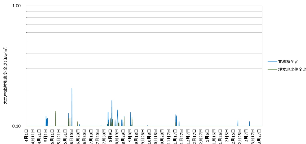
図 3-2-2 (2) 大気中放射能濃度(全 \beta )の経時変化(令和2年4月～令和3年3月)
