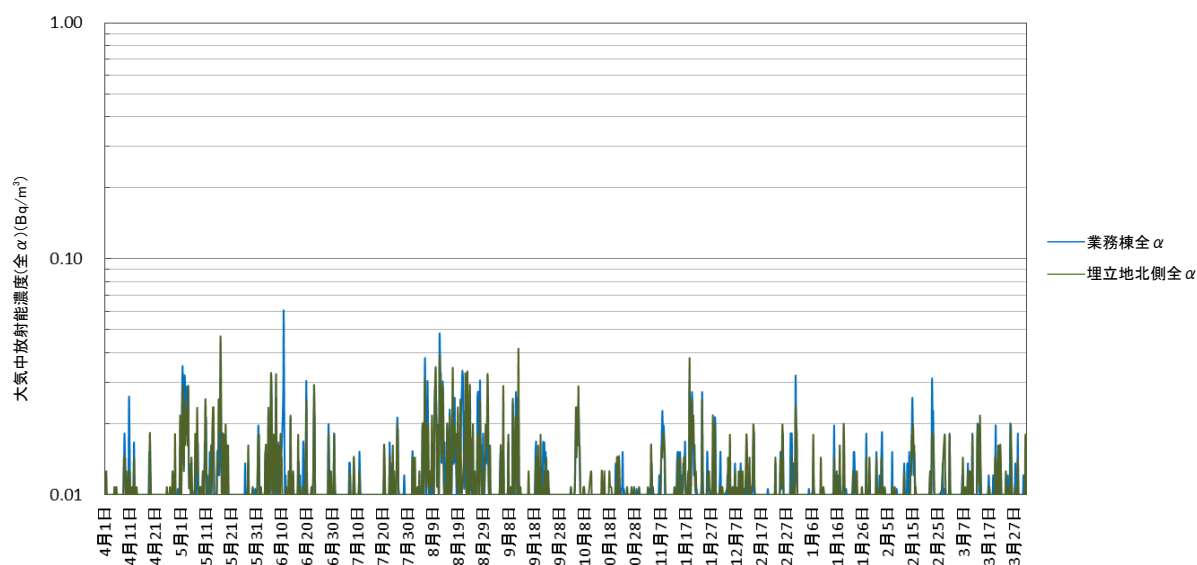
図 3-2-2 (1) 大気中放射能濃度(全 \alpha )の経時変化(令和2年4月～令和3年3月)
