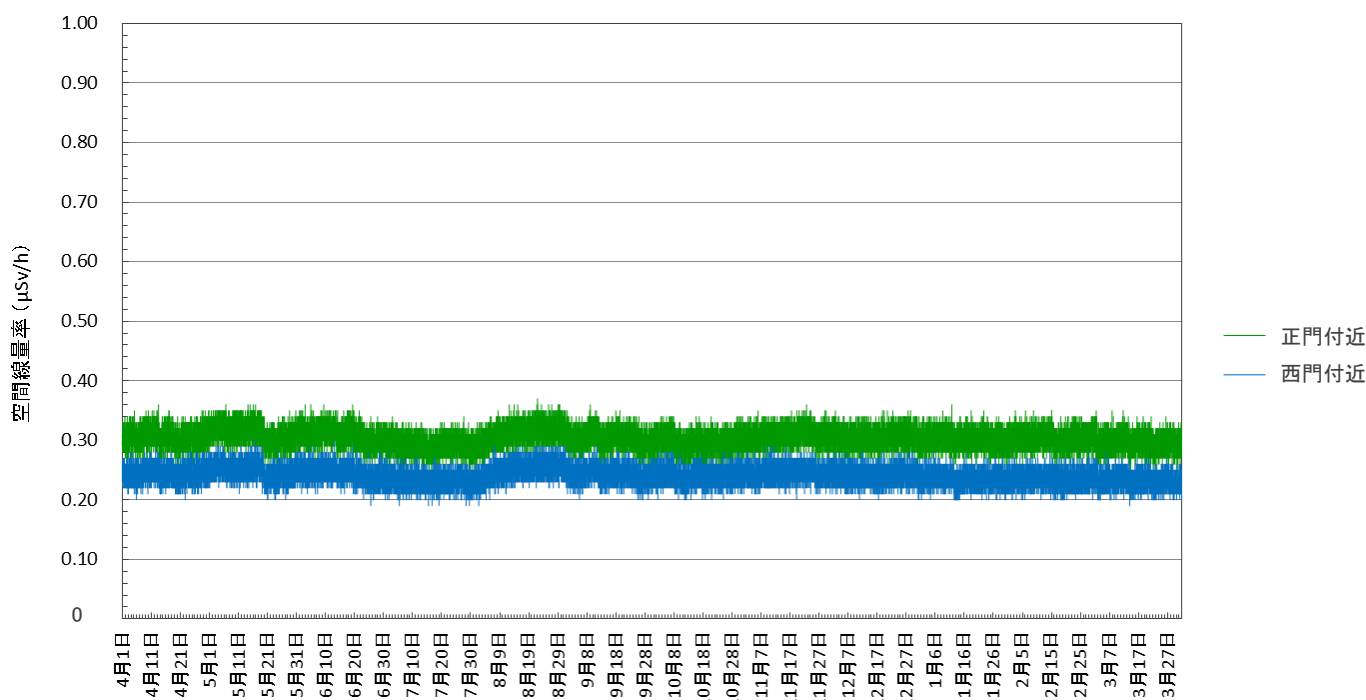
図 3-3-2 空間線量率(連続測定)の経時変化 (令和2年4月～令和3年3月)
