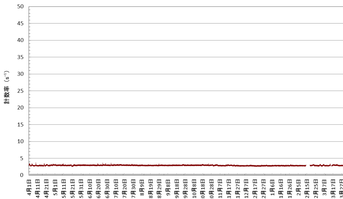
図 3-1-2 地下水中の放射能濃度(連続測定)の経時変化(令和2年4月～令和3年3月)
