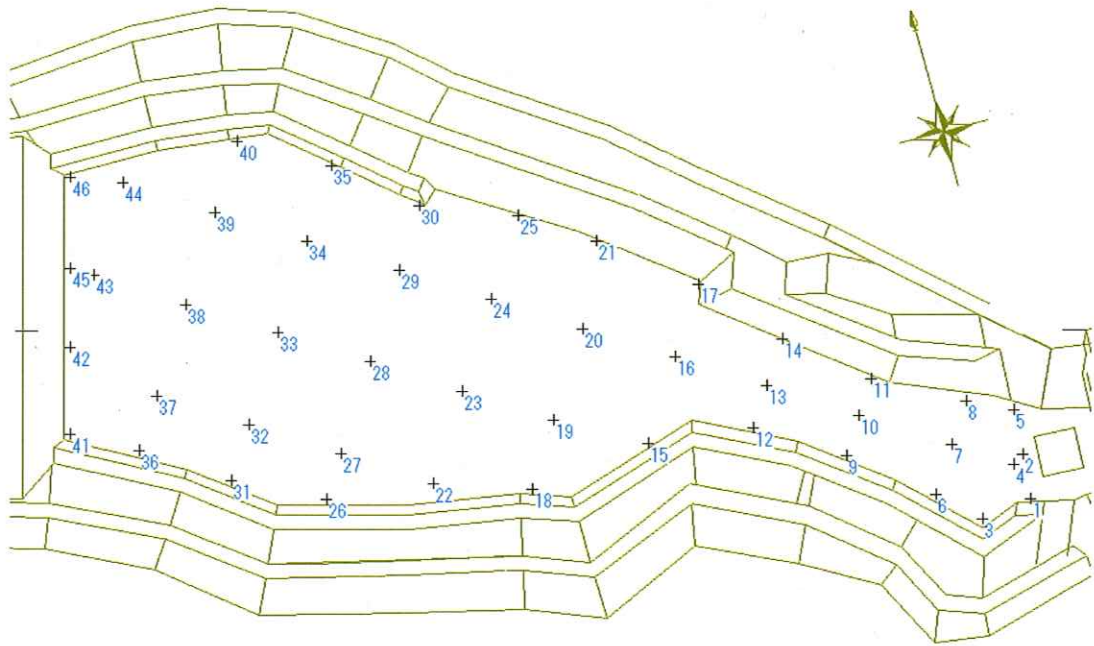
図-2.3 電極配置平面図
