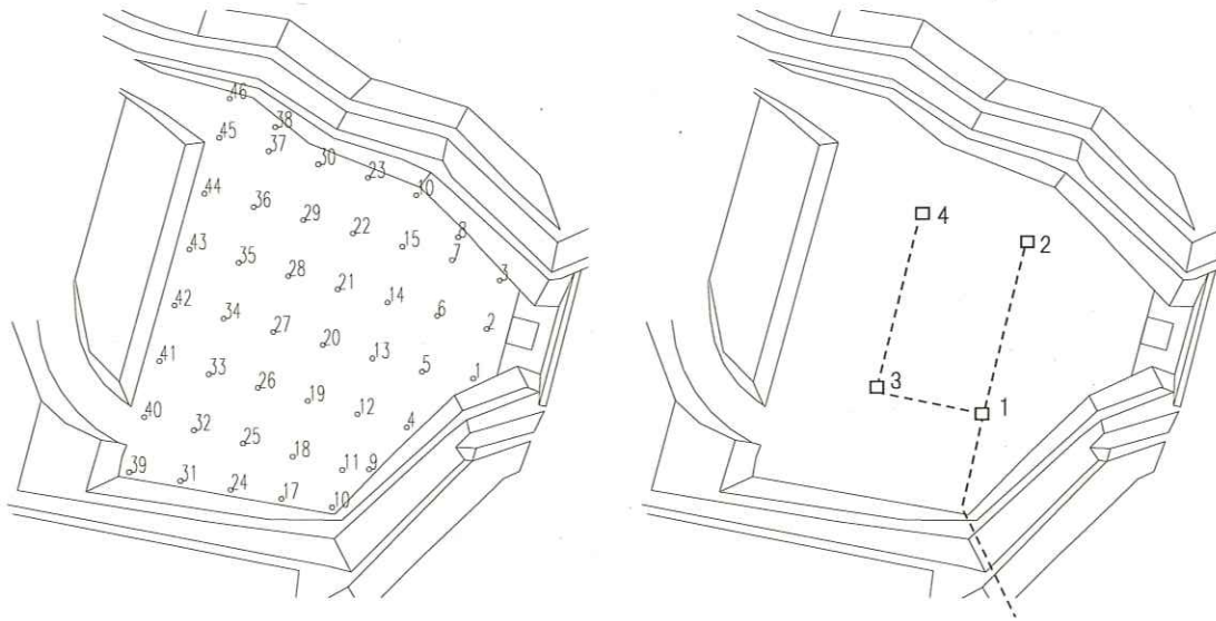
(検知電極配置図)
