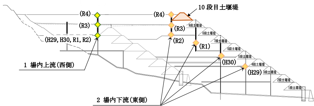
埋立ガスの調査位置(断面図)
