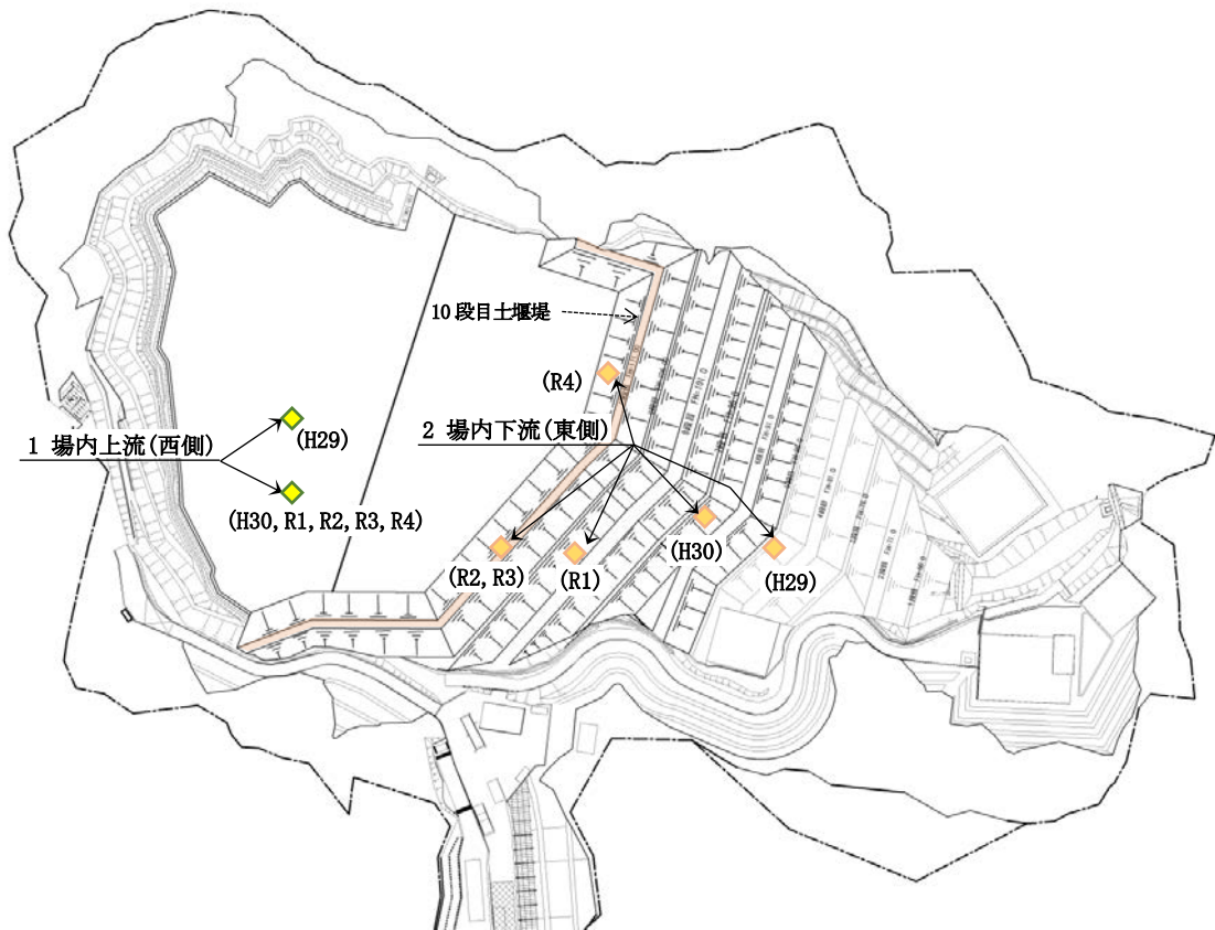
埋立ガスの調査位置(平面図)
