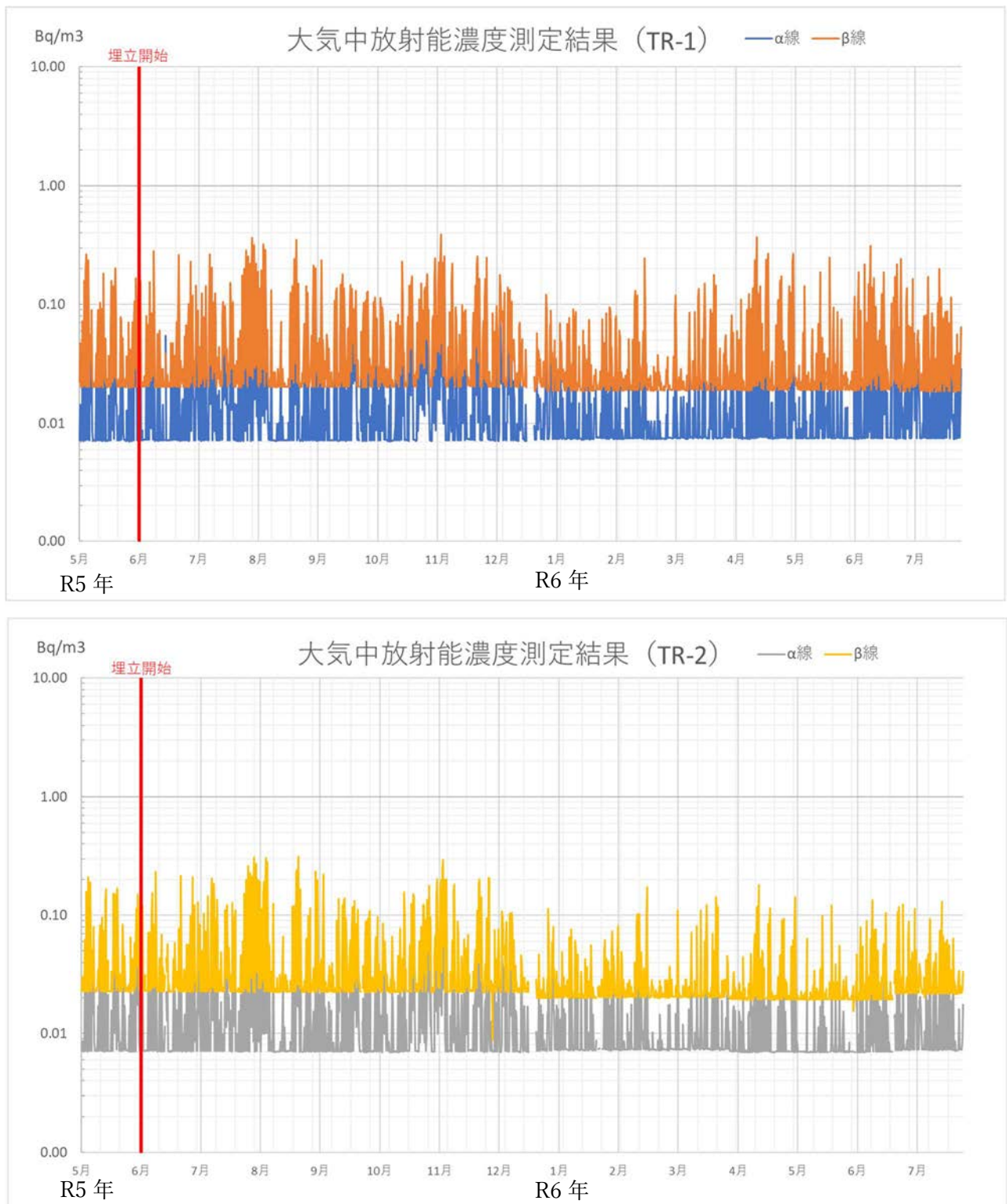
図 4.6 大気中放射能濃度測定結果
