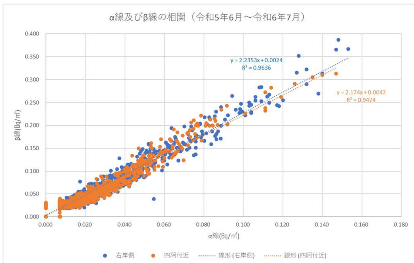
図 4.7 大気中放射能濃度測定結果( \beta/\alpha 比)
