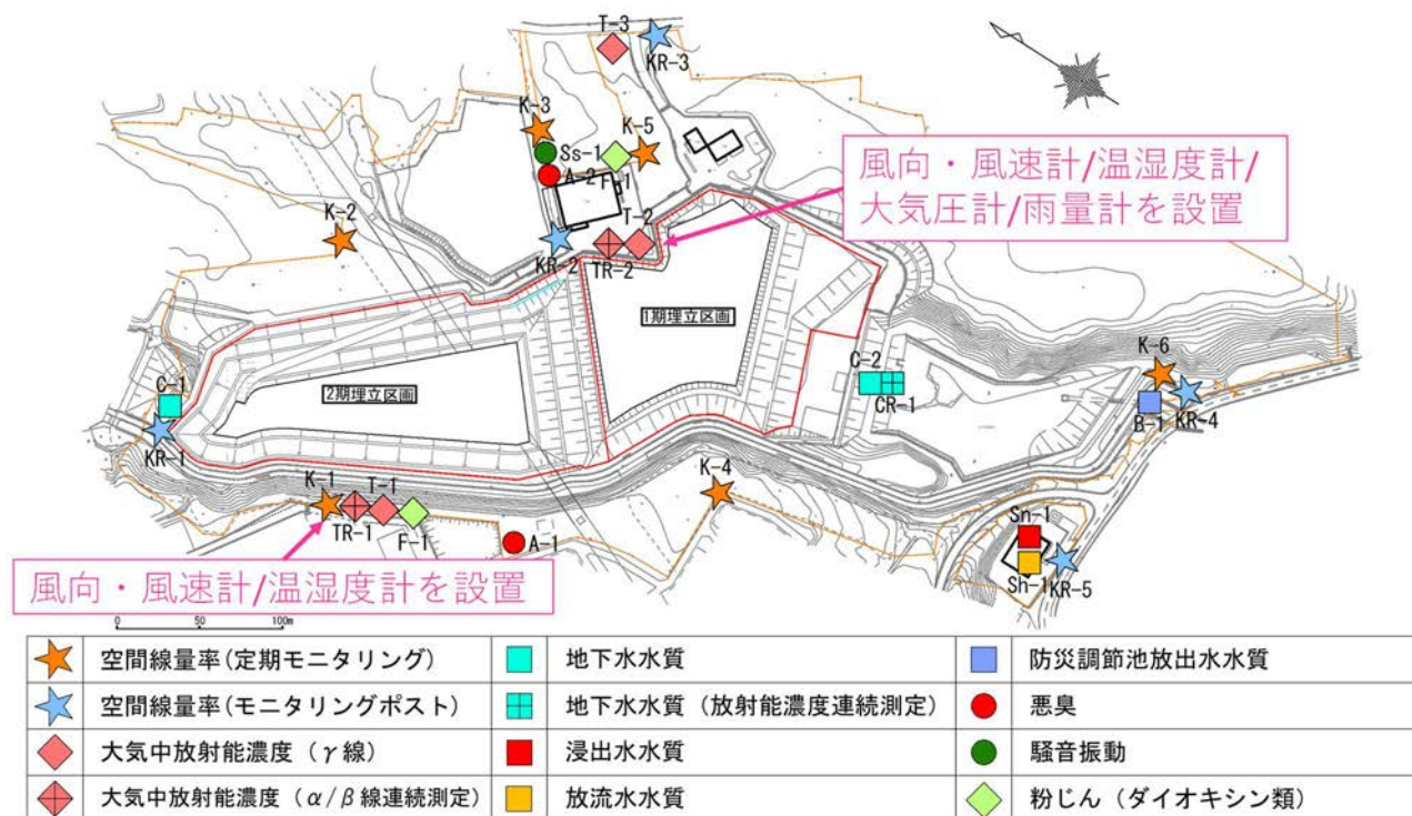
図 3.1 埋立処分場内の調査位置
