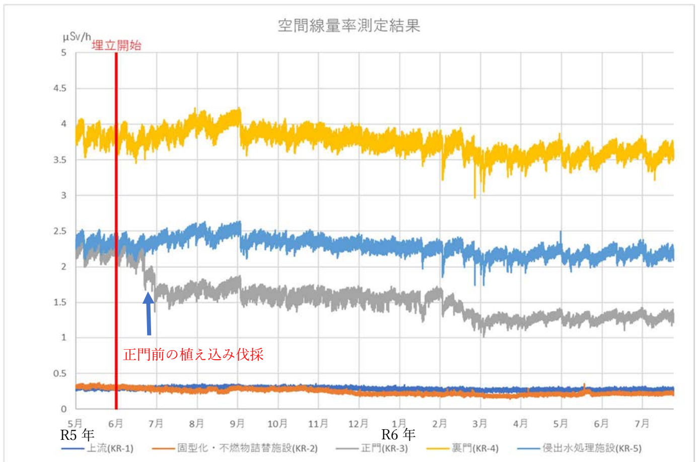
図 4.4 モニタリングポストの空間線量率の調査結果
