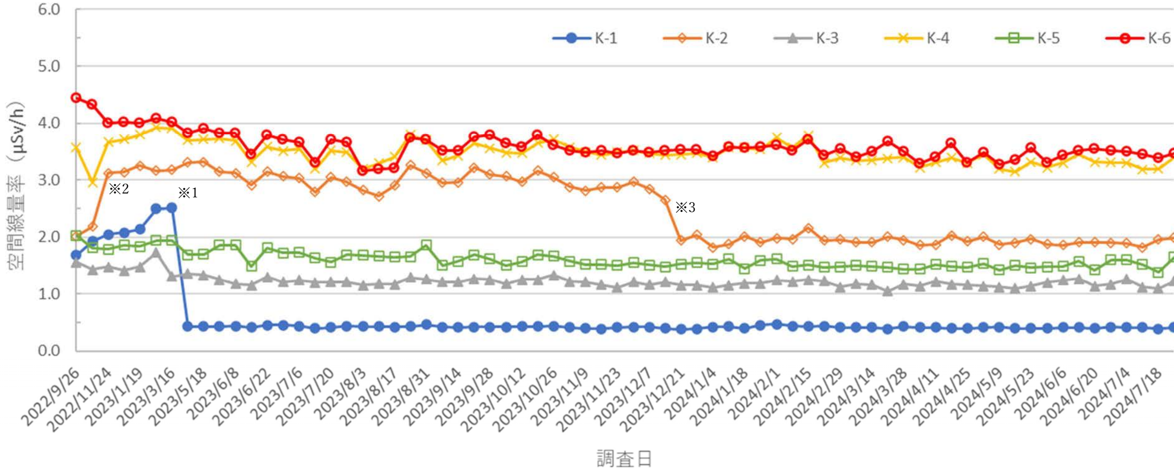
図 4.3 敷地境界の空間線量率の調査結果
