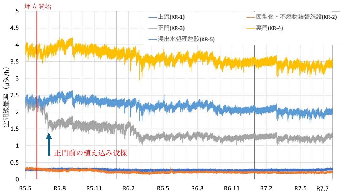
図 4.4 モニタリングポストの空間線量率の調査結果
