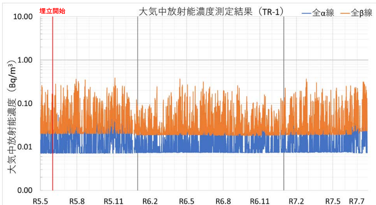
図 4.6 大気中放射能濃度測定結果(TR-1)
