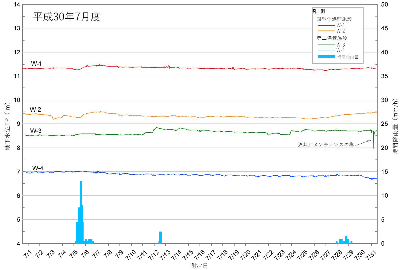
図-3 地下水位測定結果及び時間降雨量（平成30年7月度）
