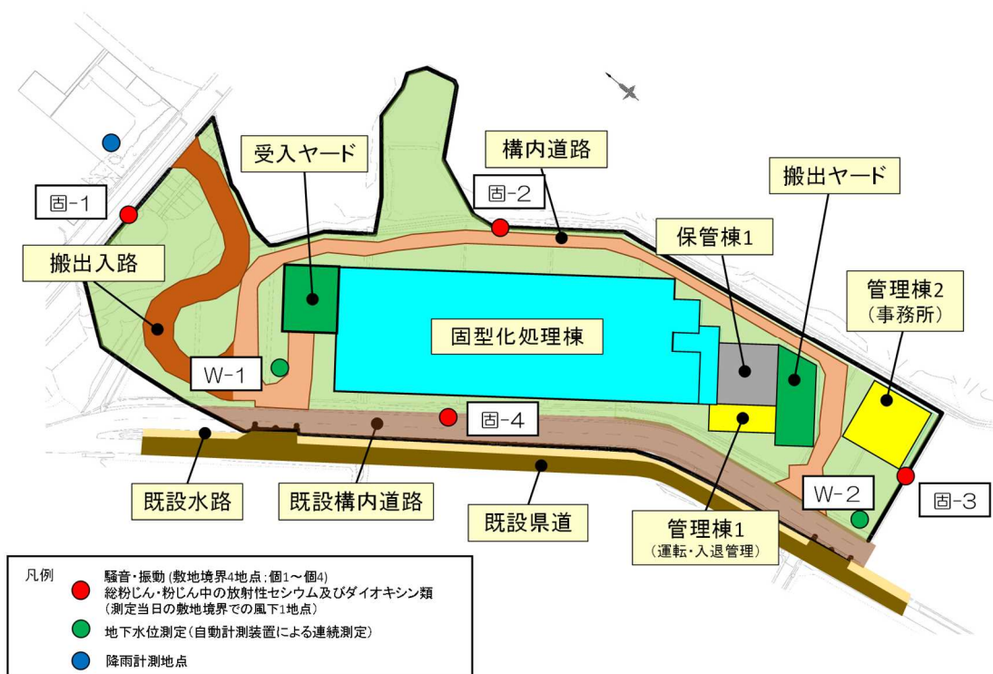
図-4 固型化処理施設における施設配置計画図
