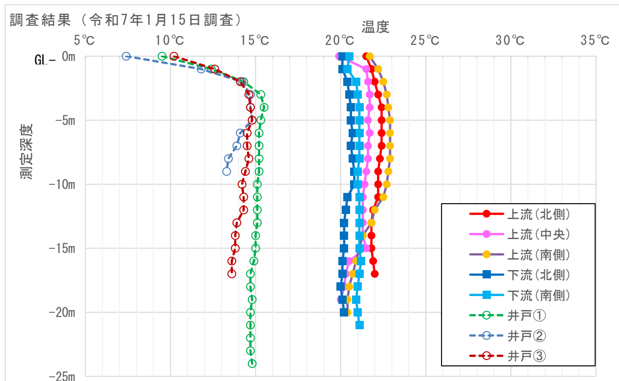
図 2-7-2 (2) 埋立地内部温度、既設井戸孔内温度の調査結果
