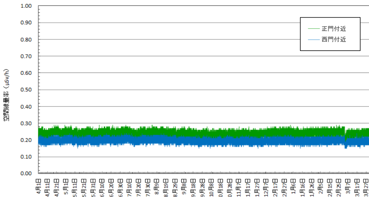
図 3-3-2 空間線量率(連続測定)の経時変化 (令和6年4月～令和7年3月)
