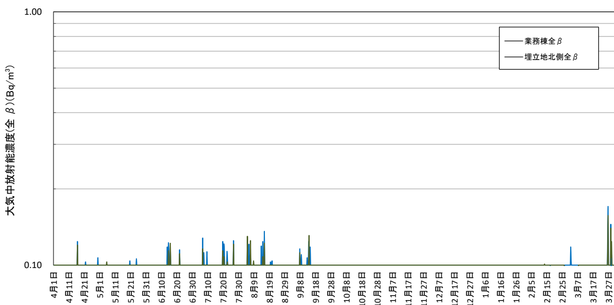
図 3-2-2 (2) 大気中放射能濃度(全 \beta )の経時変化(令和6年4月～令和7年3月)
