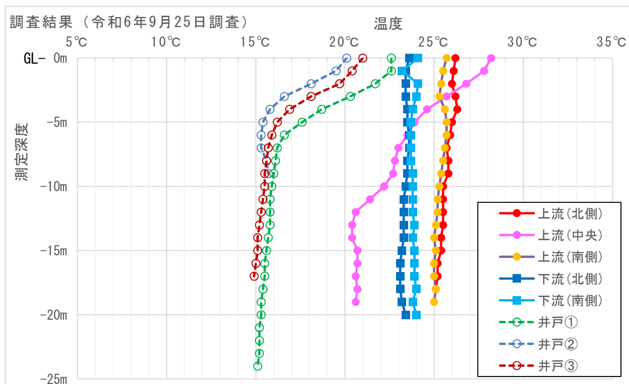
図 2-7-2 (1) 埋立地内部温度、既設井戸孔内温度の調査結果
