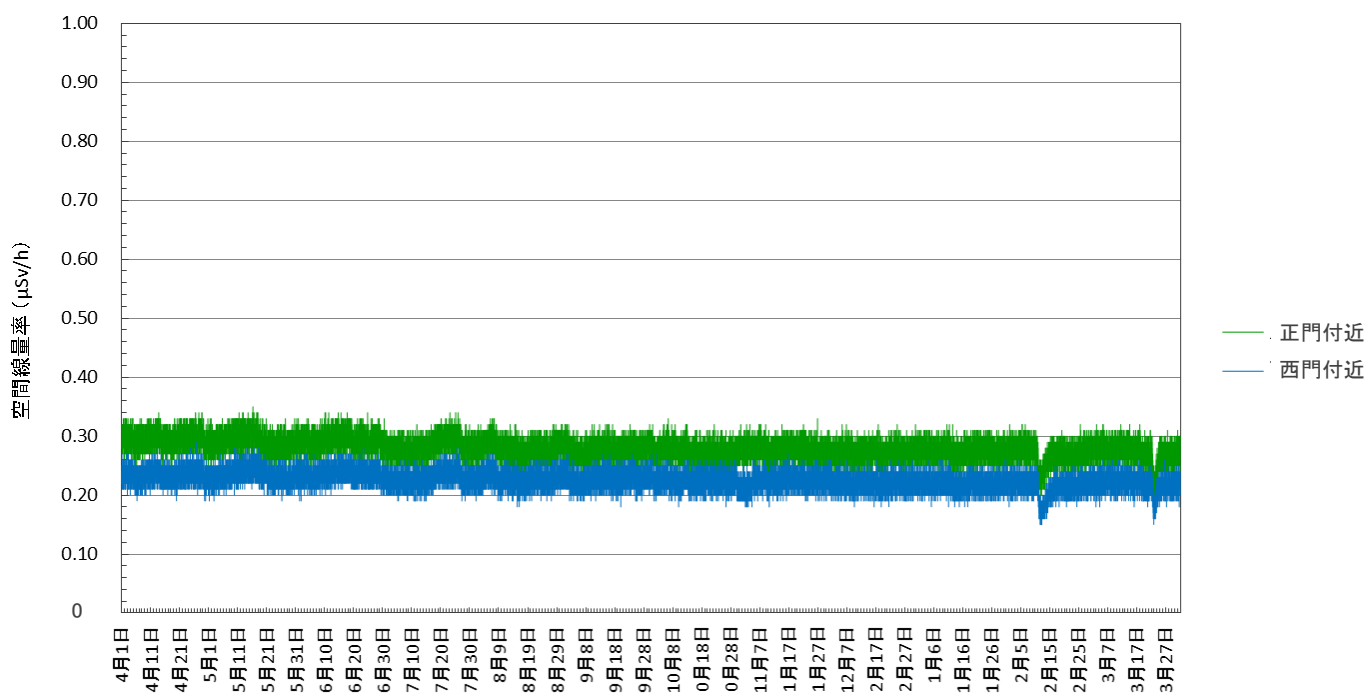
図 3-3-2 空間線量率(連続測定)の経時変化 (令和3年4月～令和4年3月)
