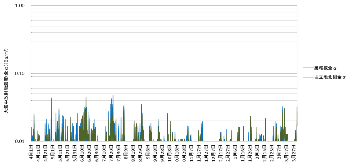
図 3-2-2 (1) 大気中放射能濃度(全 \alpha )の経時変化(令和3年4月～令和4年3月)
