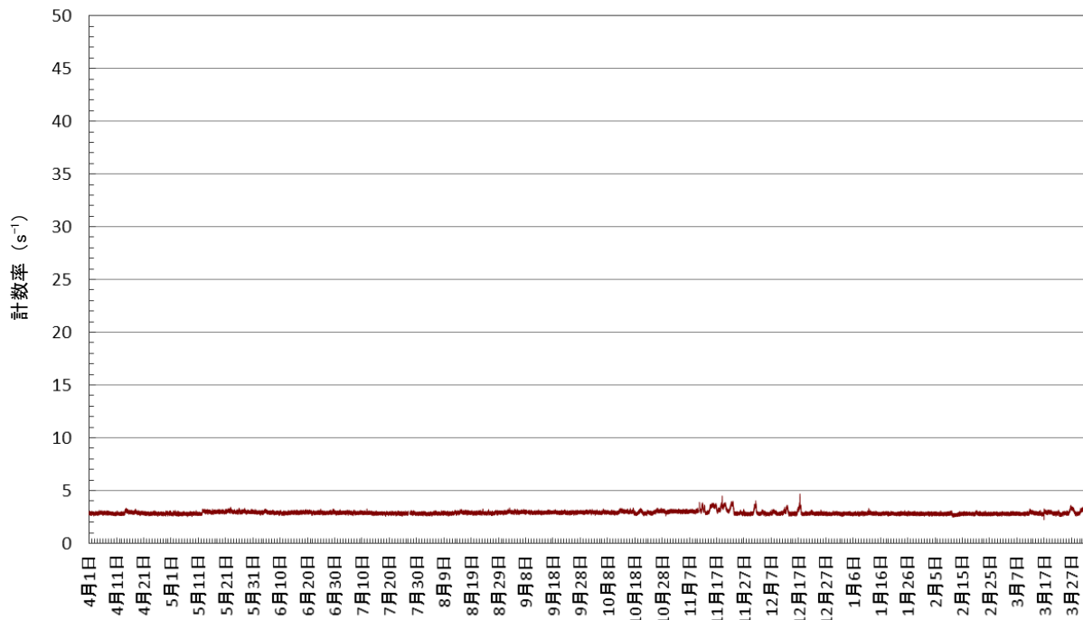
図 3-1-2 地下水中の放射能濃度(連続測定)の経時変化(令和3年4月～令和4年3月)
