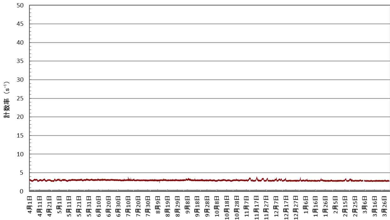
図 3-1-2 地下水中の放射能濃度(連続測定)の経時変化(令和5年4月～令和6年3月)
