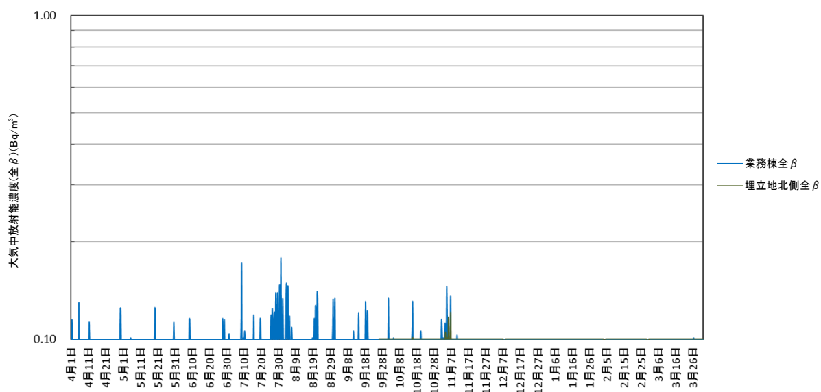
図 3-2-2 (2) 大気中放射能濃度(全β)の経時変化(令和5年4月～令和6年3月)
