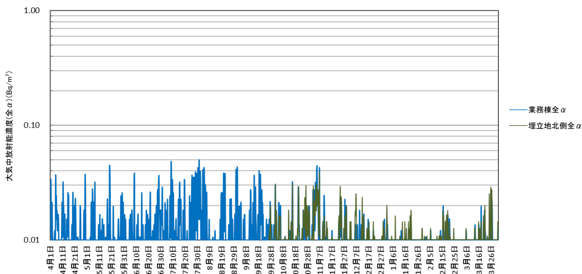
図 3-2-2 (1) 大気中放射能濃度(全α)の経時変化(令和5年4月～令和6年3月)
